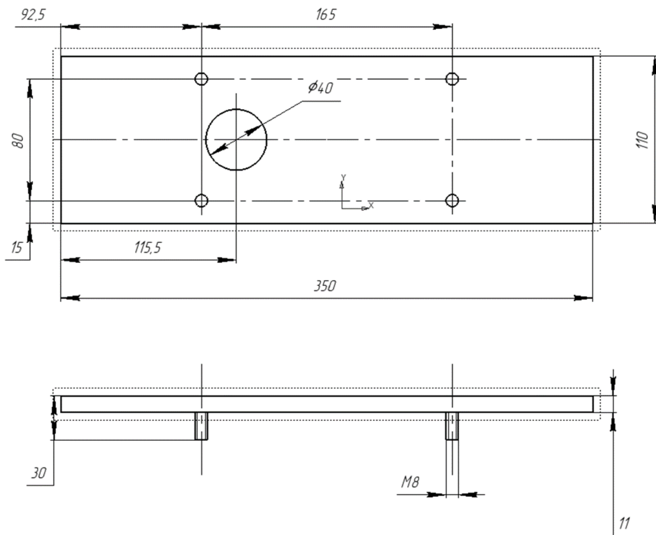
Рисунок А.7 – Эскиз габаритного чертежа АЛВР.741134.006ГЧ подставки антенны локомотивной МІМО
