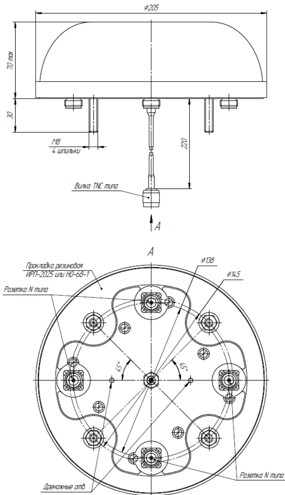
Рисунок А.6 – Эскиз габаритного чертежа АЛВР.464656.014ГЧ антенны локомотивной АЛ4/800-3400/ММО/4x4/Н
